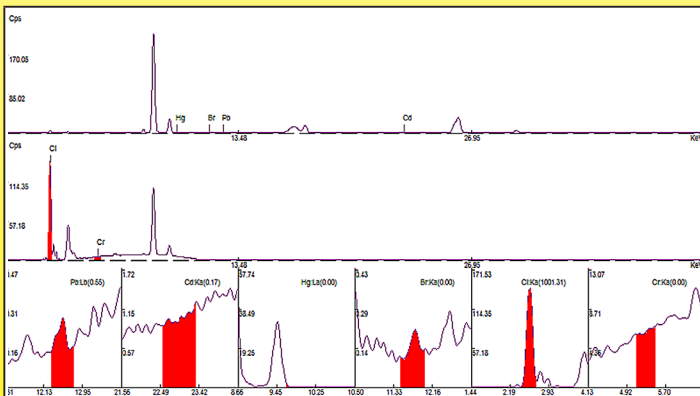
Espectrograma RoHS de una lámina de silicona reforzada con fibra de vidrio (Laboratorio Ultiheat)
